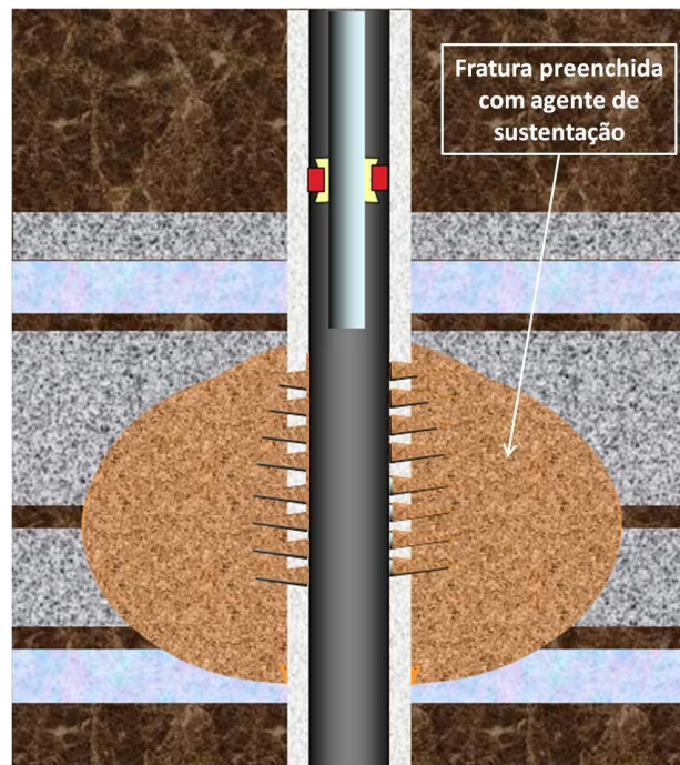
Figura 2.3 - Fratura preenchida pelo agente de sustentação após término da operação (Fonte: Elaboração própria)
