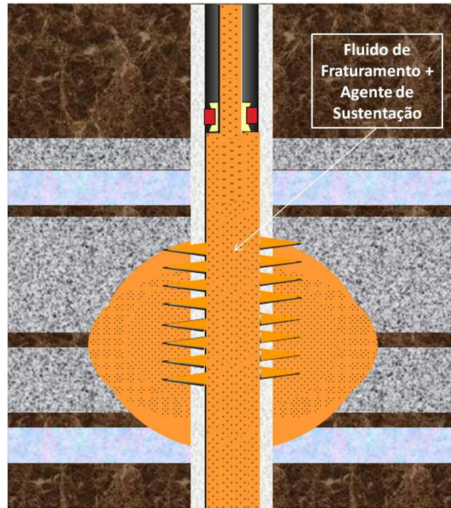
Figura 2.2 - Fratura aberta durante bombeio do fluido de fraturamento mais agente de sustentação (Fonte: Elaboração própria)
