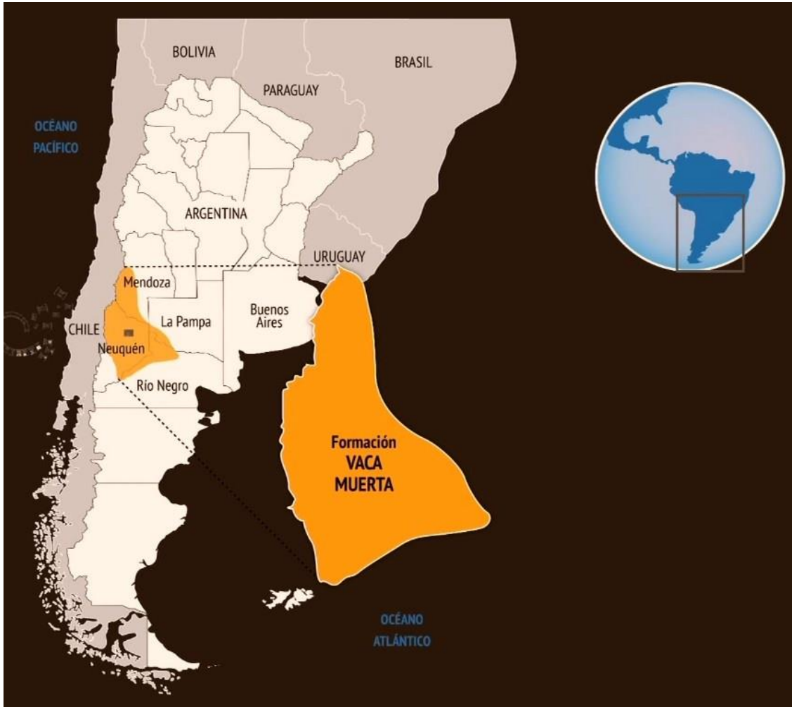
Figura 7.3 Mapa da Formação de Vaca Muerta
