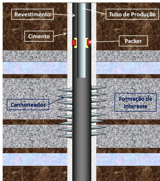
Figura 2.1 - Representação de um poço pronto para ser fraturado (Fonte: Elaboração própria)
